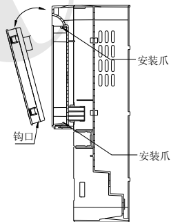
图 3-3 操作键盘的安装示意图
