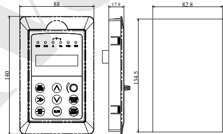
图 2-8 键盘安装盒外形及开孔尺寸
