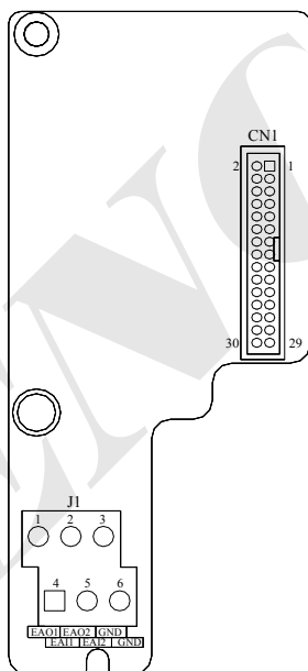
图 G-1 EN-AI1 外形尺寸图
