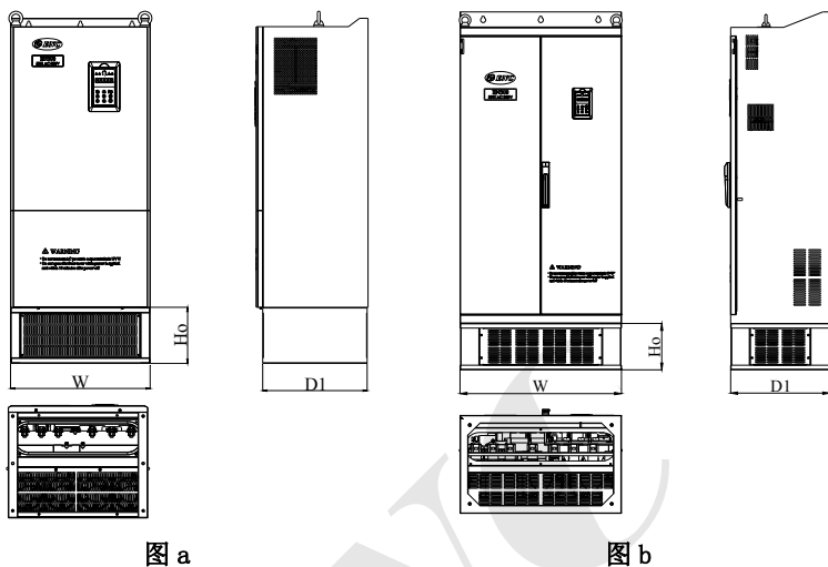
图 2-6 底座外形图
